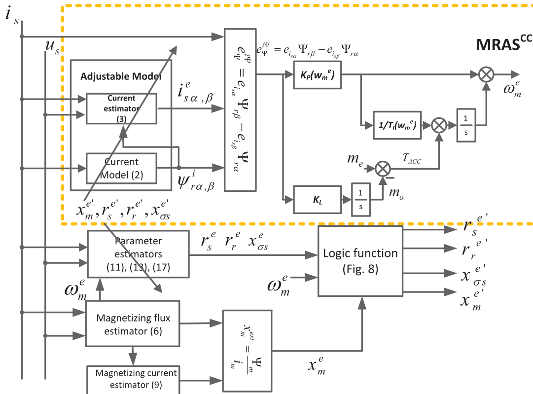
Fig. 7. Universal estimator scheme
